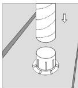
После установки гибкого воздуховода на корпус: 1. Укрепите с помощью ленты ALU 2. Закрепите с помощью хомутов
